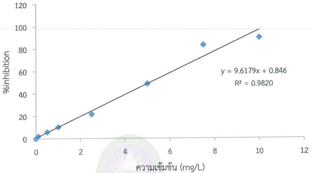
ภาพที่ ค-2 กราฟสมการในการคำนวณหาร้อยละการยับยั้งของสารมาตรฐานกรดแอสคอร์บิก วิธี DPPH*
