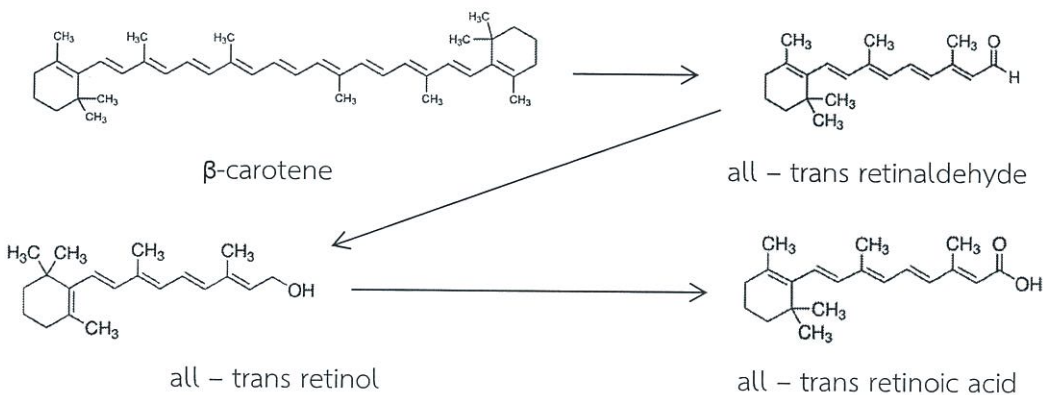
ภาพที่ 2.2 การสังเคราะห์วิตามินเอจากเบต้าแคโรทีน (อัญชญา เจนวิถีสุข, 2545)
