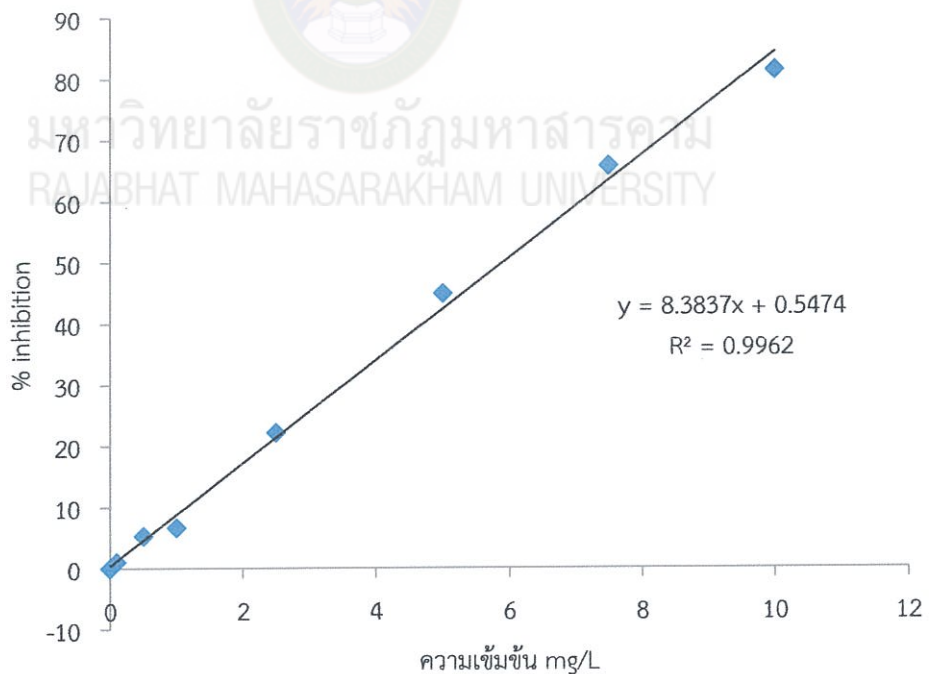
ภาพที่ ข-2 กราฟความสัมพันธ์ของสารมาตรฐานไทโรลอกที่ความเข้มข้นต่างๆ กับ %inhibition ด้วยวิธี DPPH*
