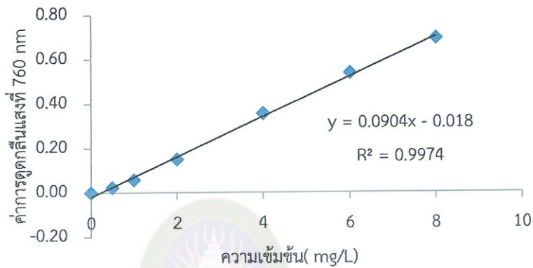
ภาพที่ 4.8 กราฟความสัมพันธ์ของสารมาตรฐานกรดแกลลิก (mg/L) ที่ความเข้มข้นต่างๆ ด้วยวิธี Folin-Ciocalteu
