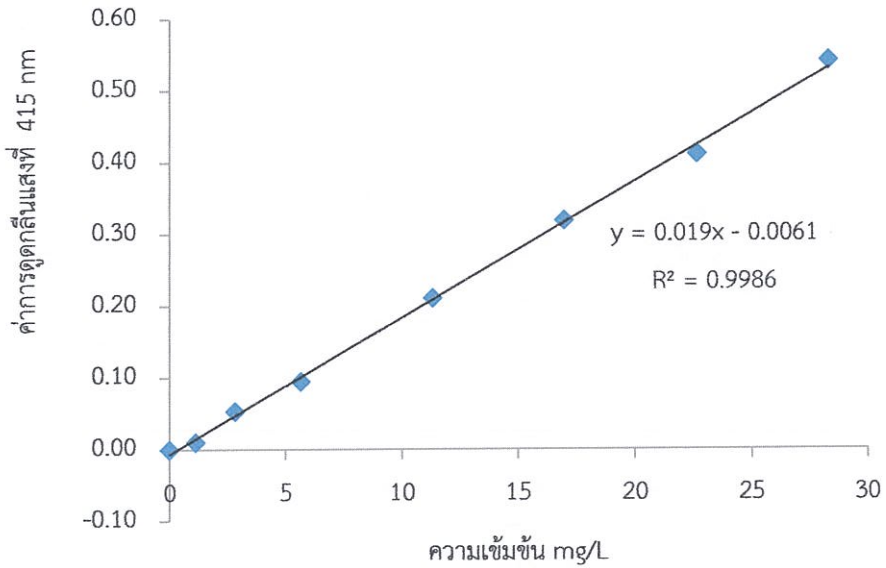
ภาพที่ ข-9 กราฟความสัมพันธ์ของสารมาตรฐานเคออลูมิเนียม (mg/L) ความเข้มข้นต่างๆ ด้วยวิธี Aluminium chloride colorimetric
