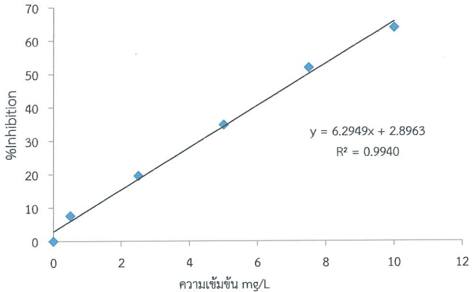
ภาพที่ ข-5 กราฟความสัมพันธ์ของสารมาตรฐานโทรลอกที่ความเข้มข้นต่างๆ กับ %inhibition ด้วยวิธี ABTS +
