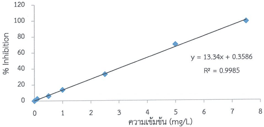
ภาพที่ ค-2 กราฟสมการในการคำนวณหาร้อยละการยับยั้งของสารมาตรฐานกรดแอสคอร์บิก วิธี ABTS •+
