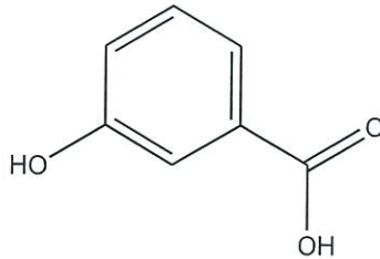
ภาพที่ 2.3 สูตรโครงสร้างของสารประกอบฟีนอลิก
