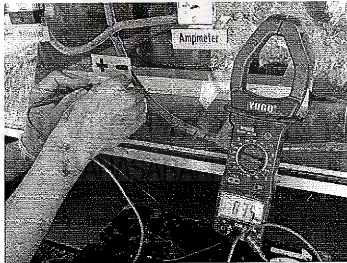
รูป ข4 ค่าแรงดันที่กังหันลผลิตได้
