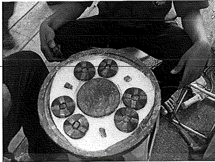
รูป ก5 ประกอบชุดขดลวด
